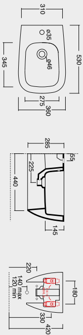
Cod. 45010101 Bidet sospeso Wunder Wunder bidet wall hung
