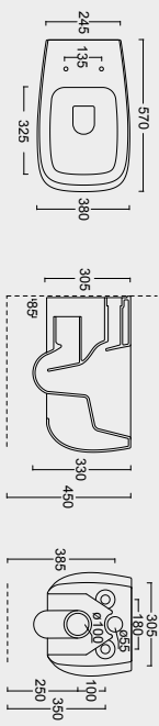
Cod. 33120101 Vaso sospeso Nur Nur WC wall hung
